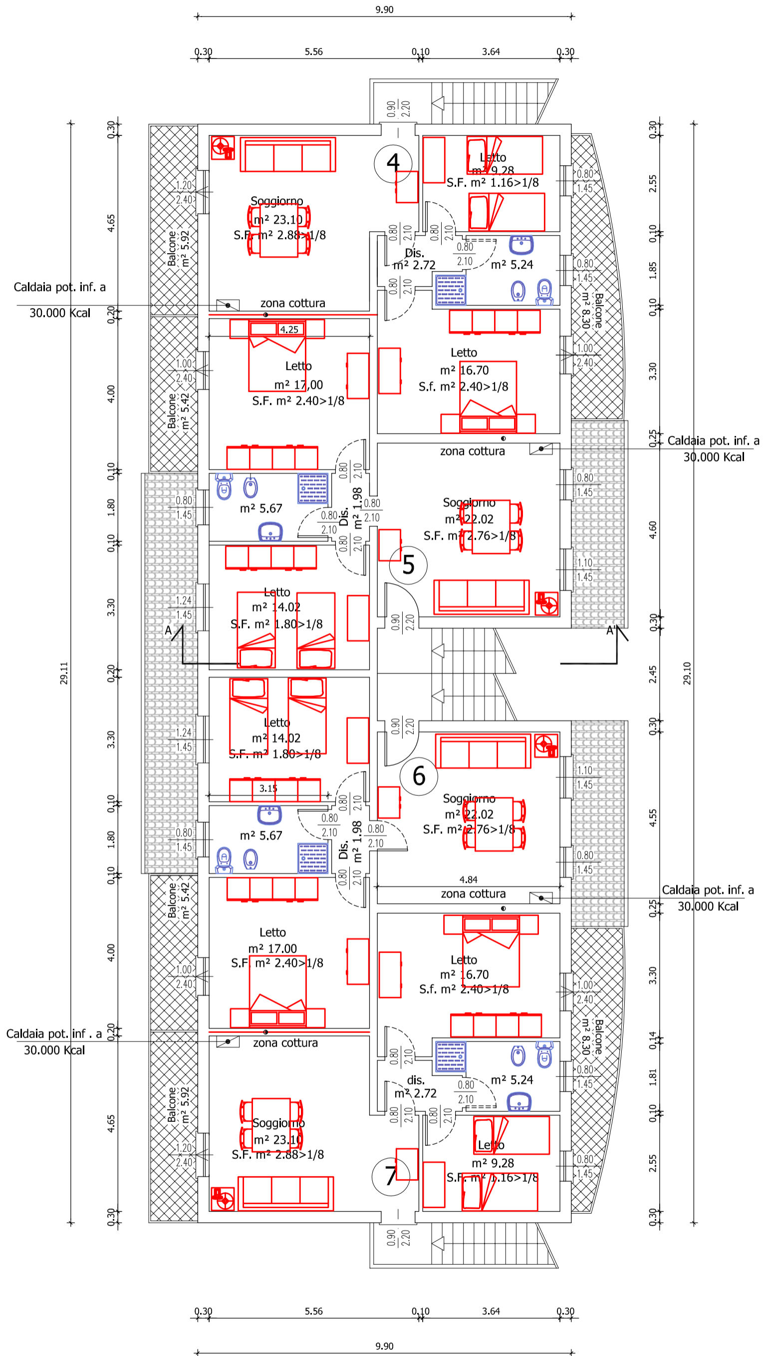
PIANTA PIANO PRIMO Scala 1:100
