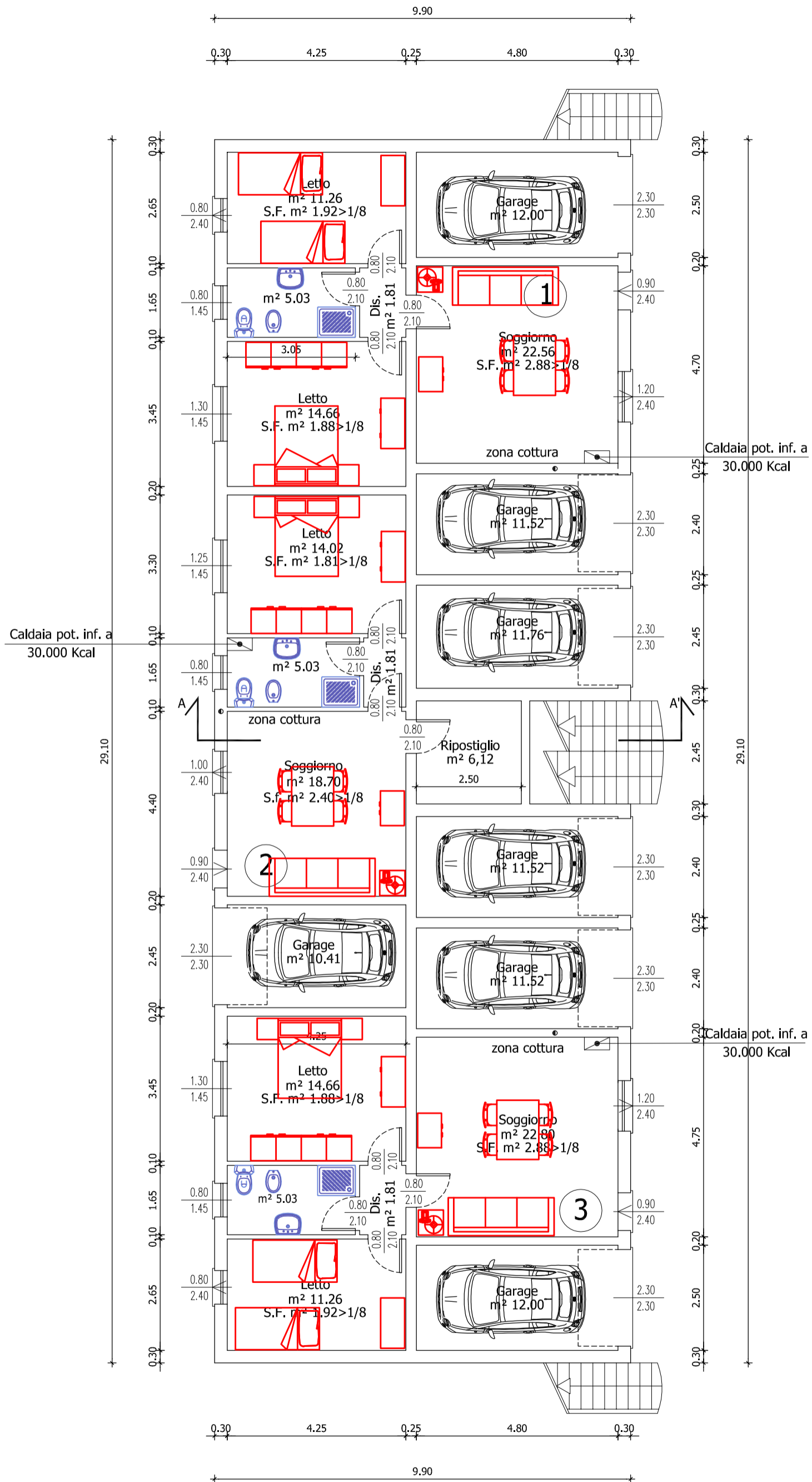
PIANTA PIANO TERRA Scala 1:100
